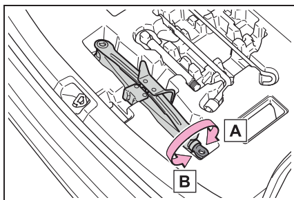
2 הוצאת את המגבה
